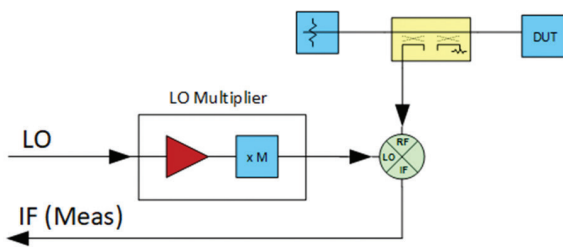
Fig. 3 - RX Extender
