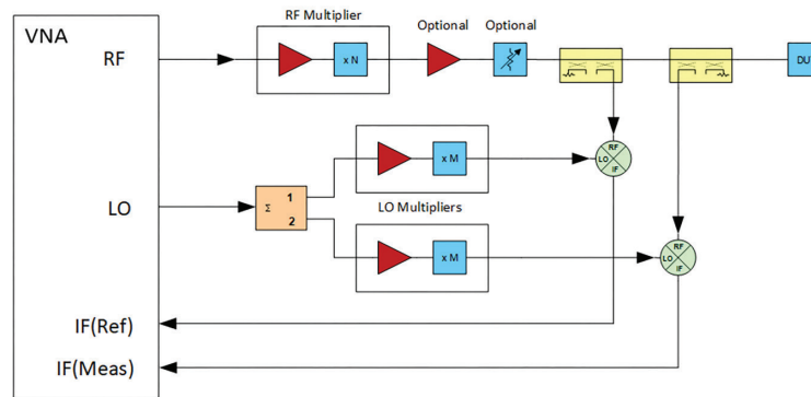
Fig. 2 - TX/RX Extender
