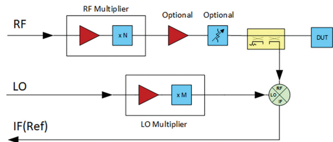
Fig. 4 - TX/REF Extender
